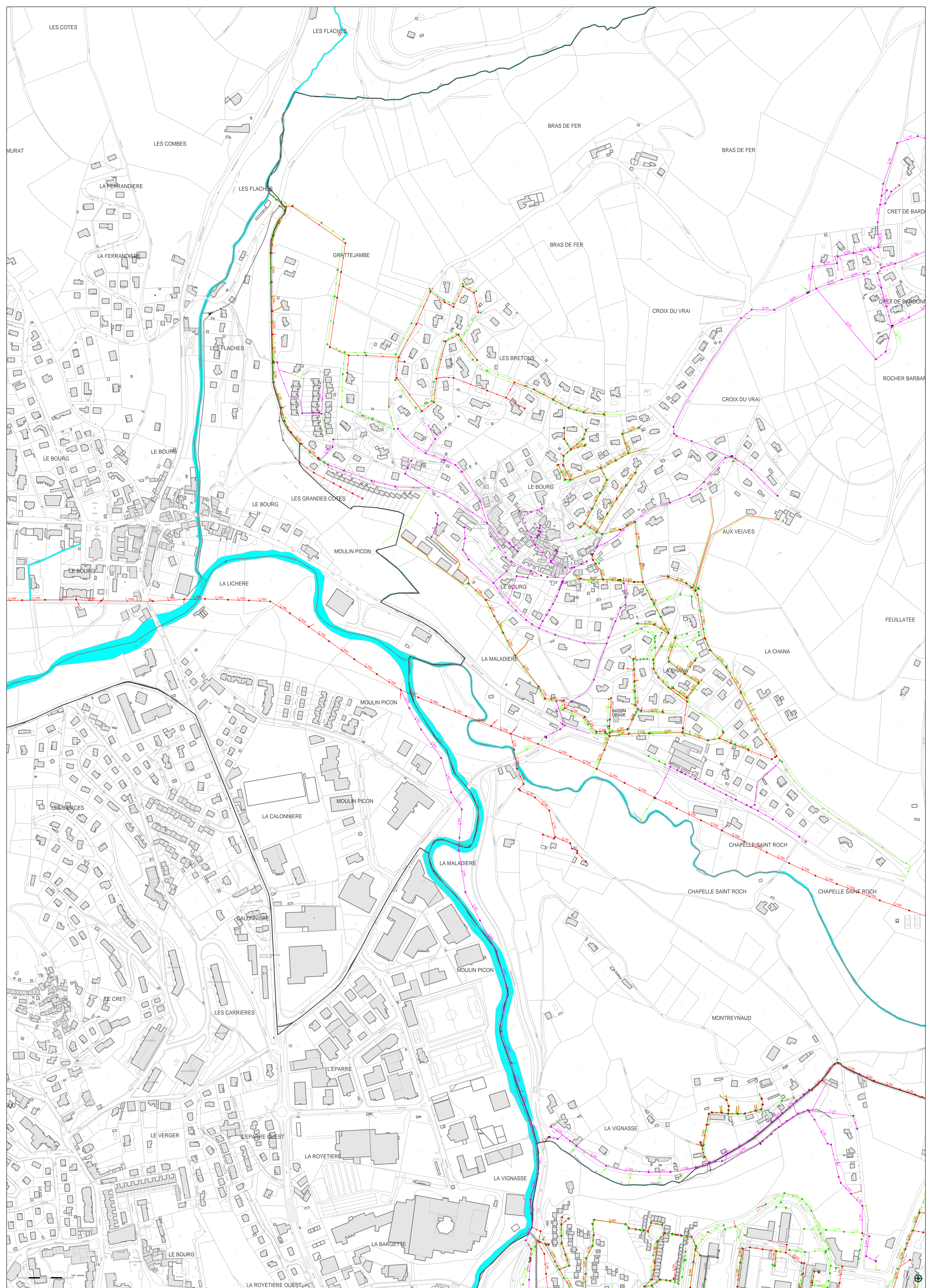
RESEAU ASSAINISSEMENT (LA TOUR-EN-JAREZ) PLAN 90 OUEST
